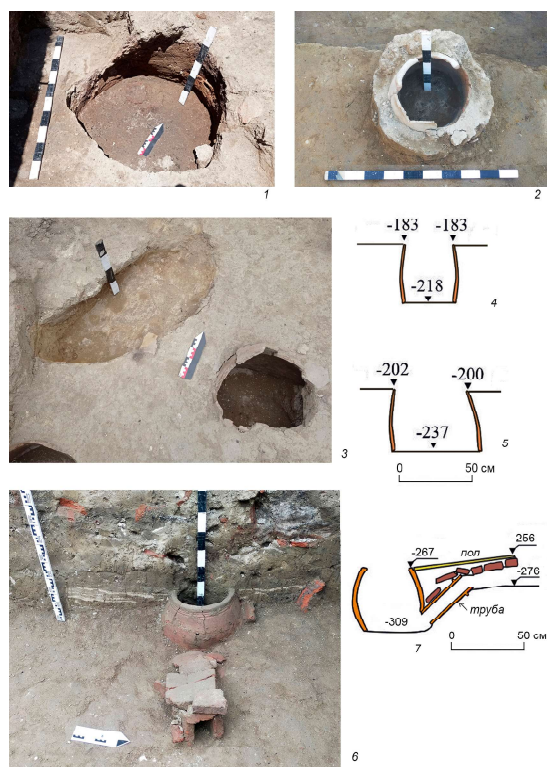
Рис. 7. Дербент. Раскоп XXXIX. Печи-корси 1–4
