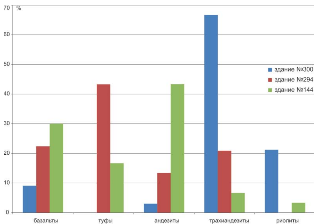
Рис. 5. Распределение вулканических пород в фундаментах акрополя.
