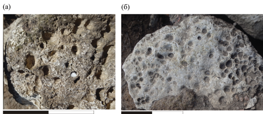
Рис. 7. Следы сверления двусторчатыми моллюсками в известняках: a – с сохранившейся раковинной. Указатель масштаба: 10 см.
