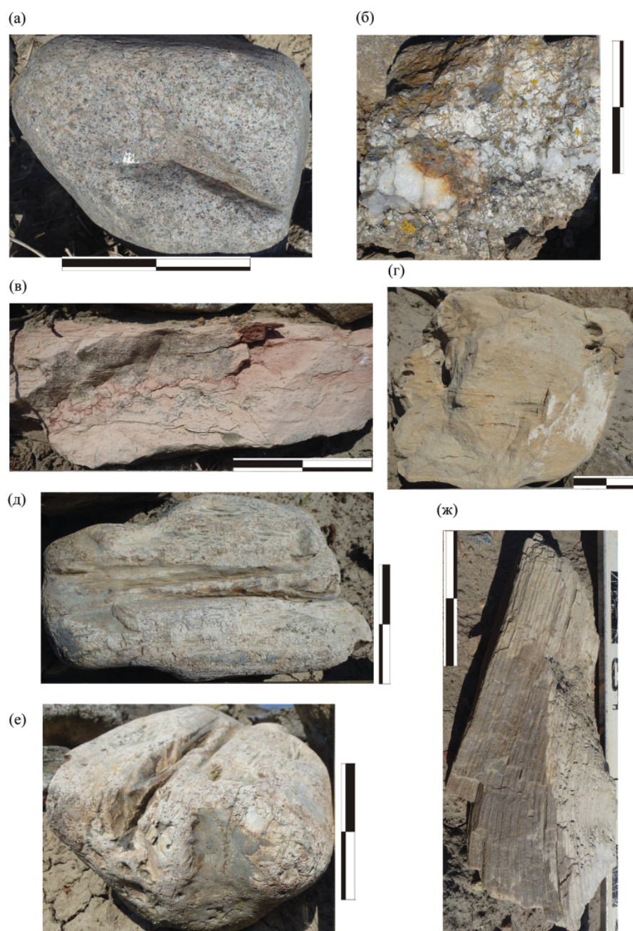
Рис. 3. Валуньы разного состава из фундаментов акрополя. Плутонические: a – розовые гранодиориты; б – кварц–полевошпатовые пегматиты; в – мергели розовые; г – песчаники; д–ж – фрагменты литифицированной древесины. Указатель масштаба: 10 см.
