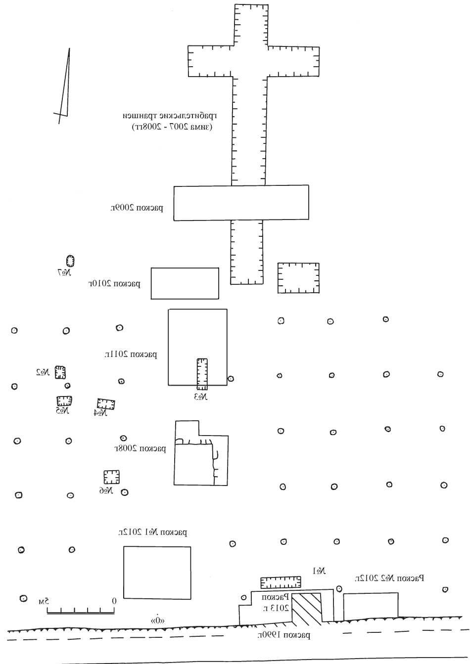
Рис. 2. Схематический план поселения Вилино (Рассадное) с грабительскими шурфами, траншеями (2007–2008 гг.) и раскопами (2008–2013 гг.) Fig. 2. Schematic plan of the settlement of Vilino (Rassadnoye) with predatory pits, 2007–2008 trenches and 2008–2013 excavations
