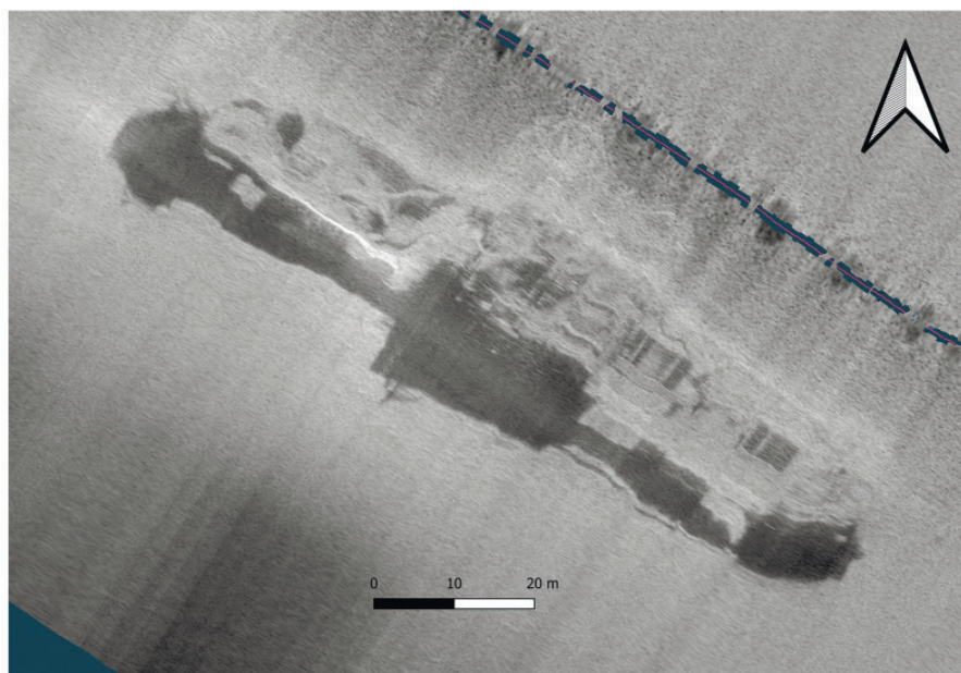
Рис. 3. Сонаграмма затонувшего судна у Нового Афона.
