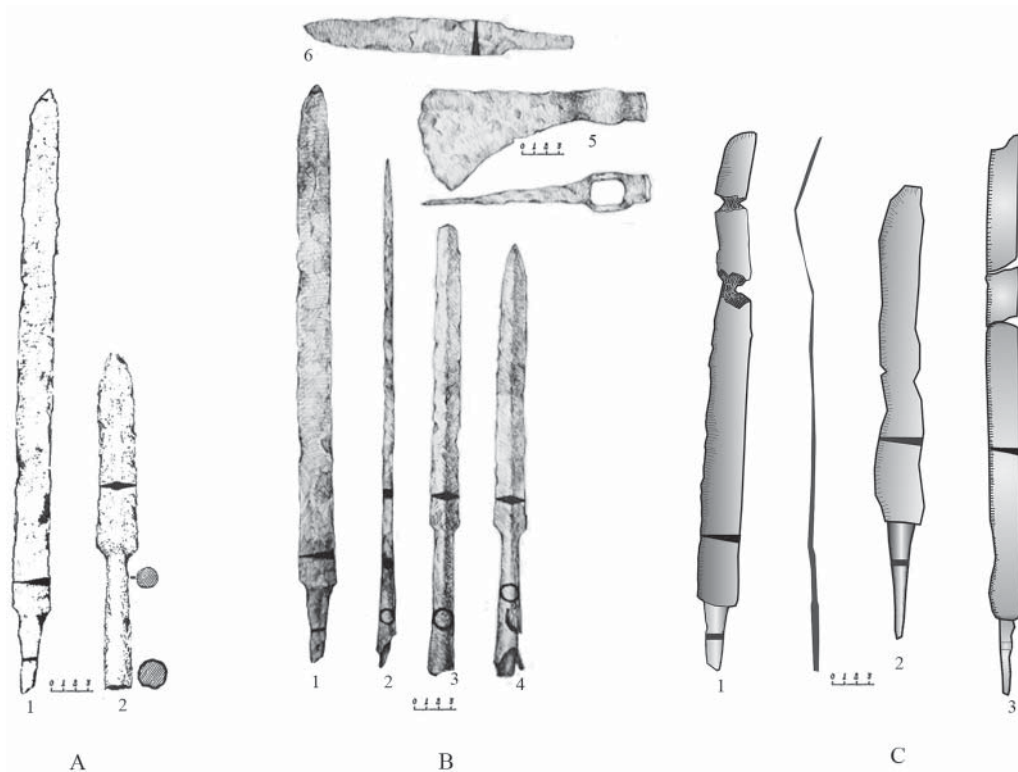
Рис. 2. Мечи из погребений села Куланьрхуа (А – Осаа-рху; В – Адеи-гуара) и Маркульского городища (С) Fig. 2. Swords from the burials in Kulanyrhua (A - Osaa-rkhu; B - Adei-guara) and Markul settlement (C)
