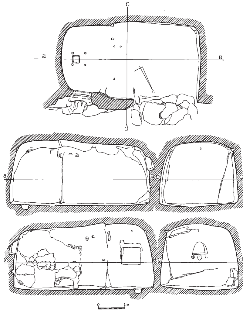
Рис. 3. Церковь на поляне Кильсе-губю. План. Разрезы
